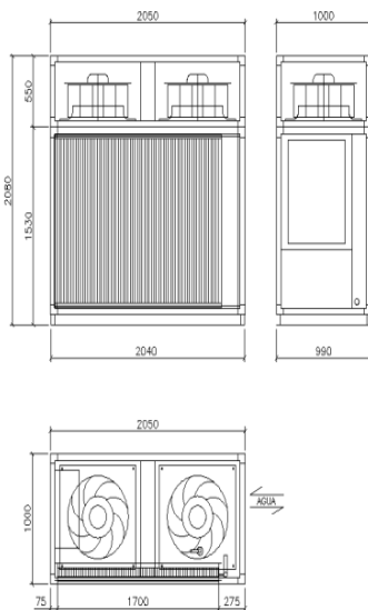
ETCB 45.1-60.1
